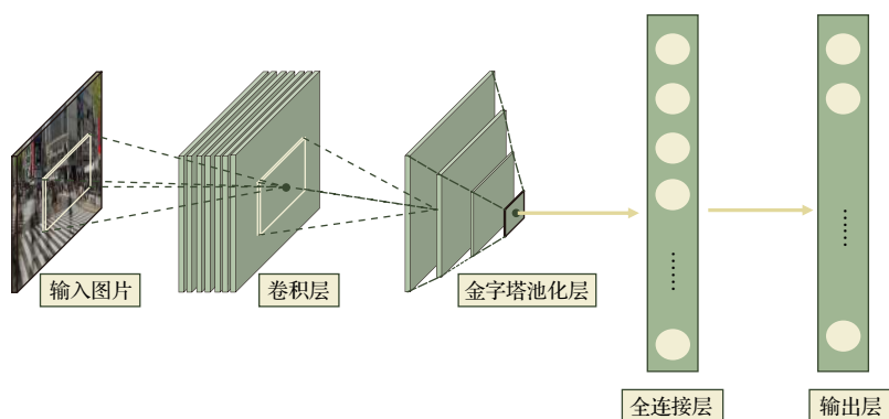
图 4 SPP-Net 结构图
