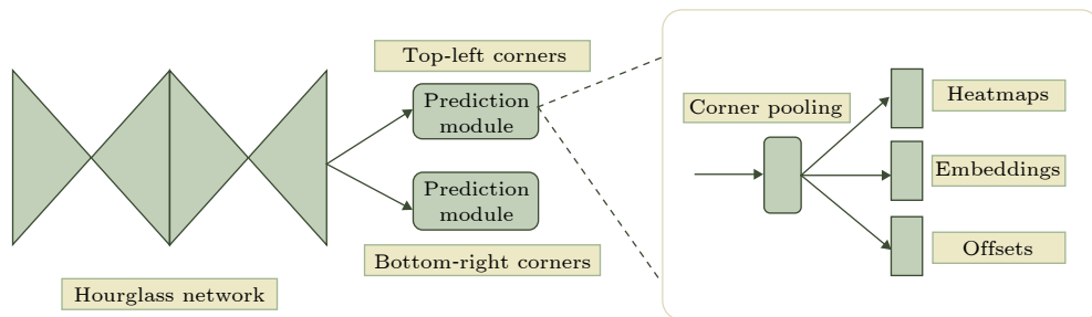
图 6 CornerNet 结构图
