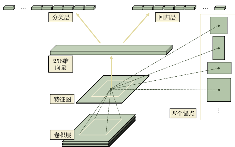
图 5 RPN 结构图
