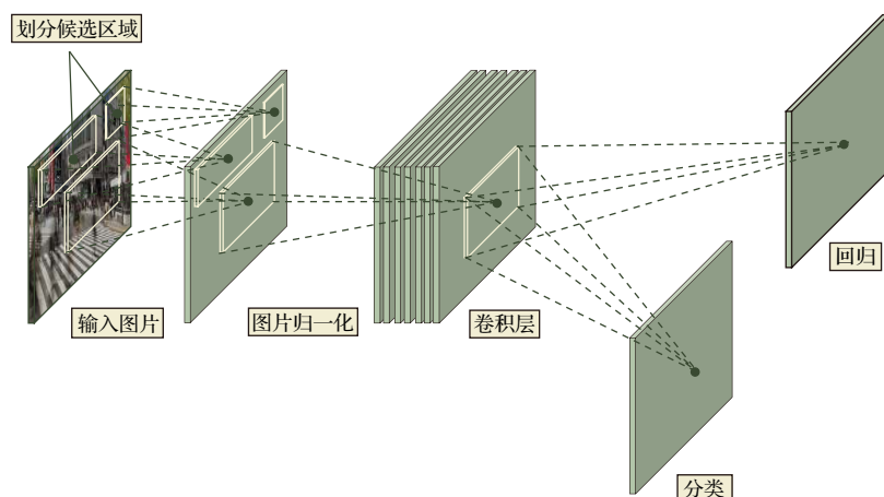
图 3 RCNN 算法流程图
