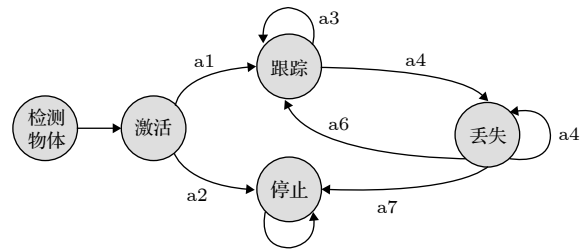
图 1 马尔科夫决策过程流程图
